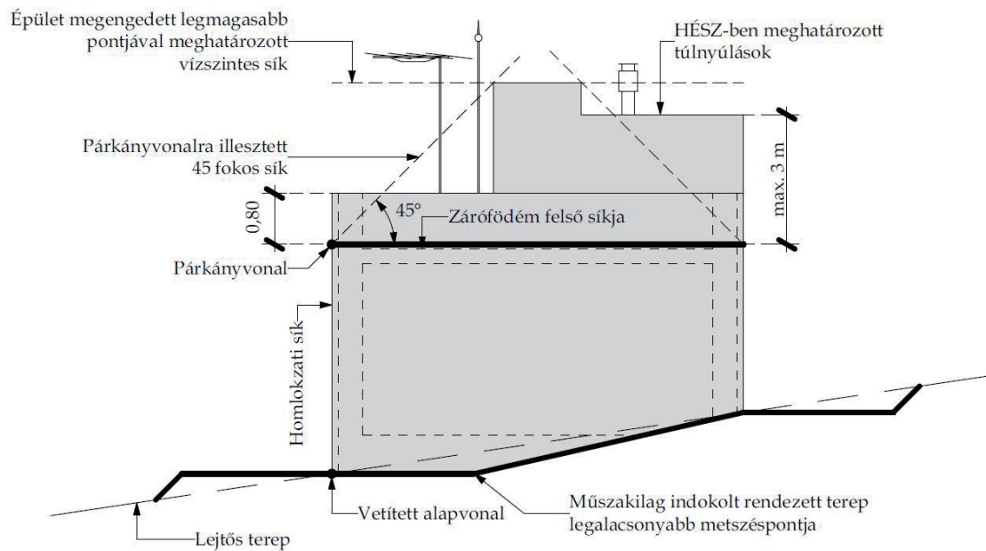
LEJTŐS TEREPEEN, LAPOSTETŐS ÉPÜLET BEÉPÍTÉSI MAGASSÁGA
