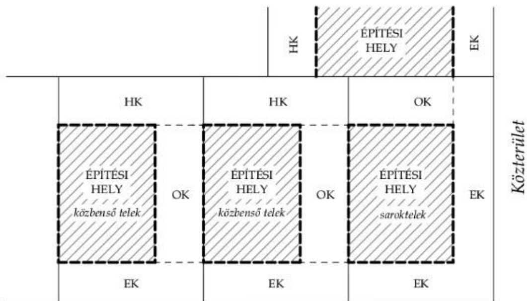
Közterület OLDALHATÁRON ÁLLÓ BEÉPÍTÉSI MÓD
