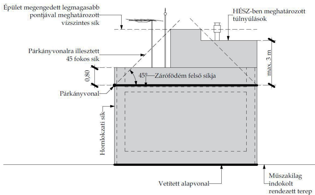
SÍK TEREPEEN, LAPOSTETŐS ÉPÜLET BEÉPÍTÉSI MAGASSÁGA
