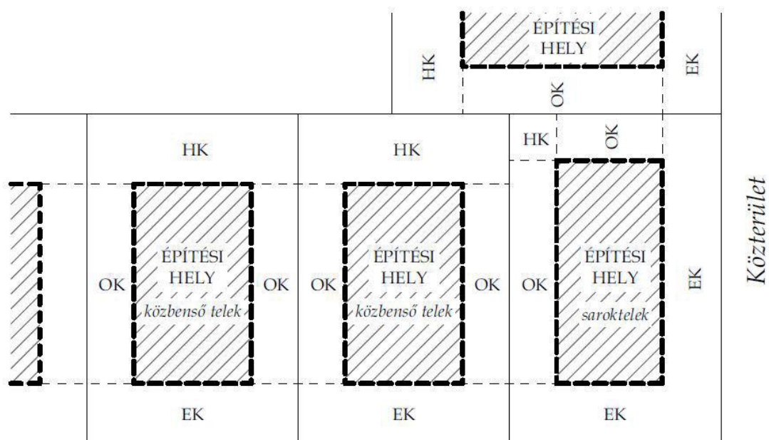
Közterület SZABADONÁLLÓ BEÉPÍTÉSI MÓD
