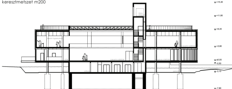
keresztmetszet m200
