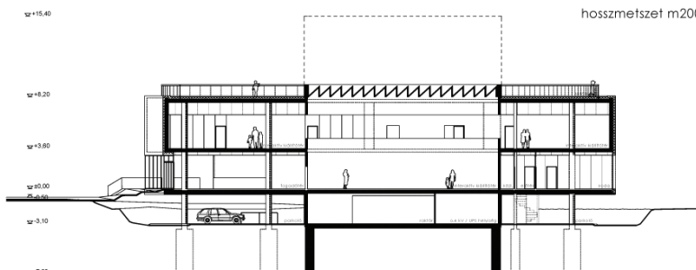
hosszmetszet m200
