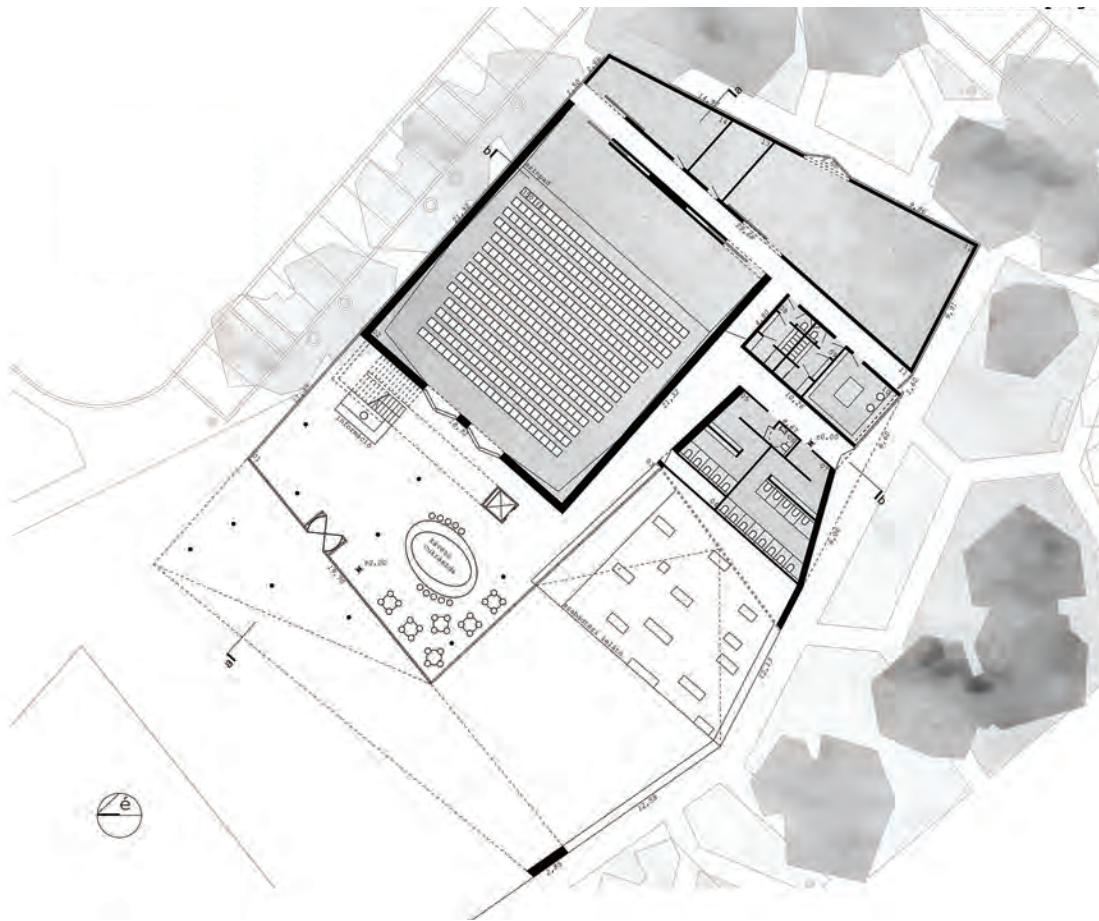
Helyszínrajz és földszinti alaprajz
