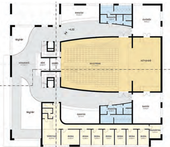
I. EMELETI ALAPRAJZ M 1:200
