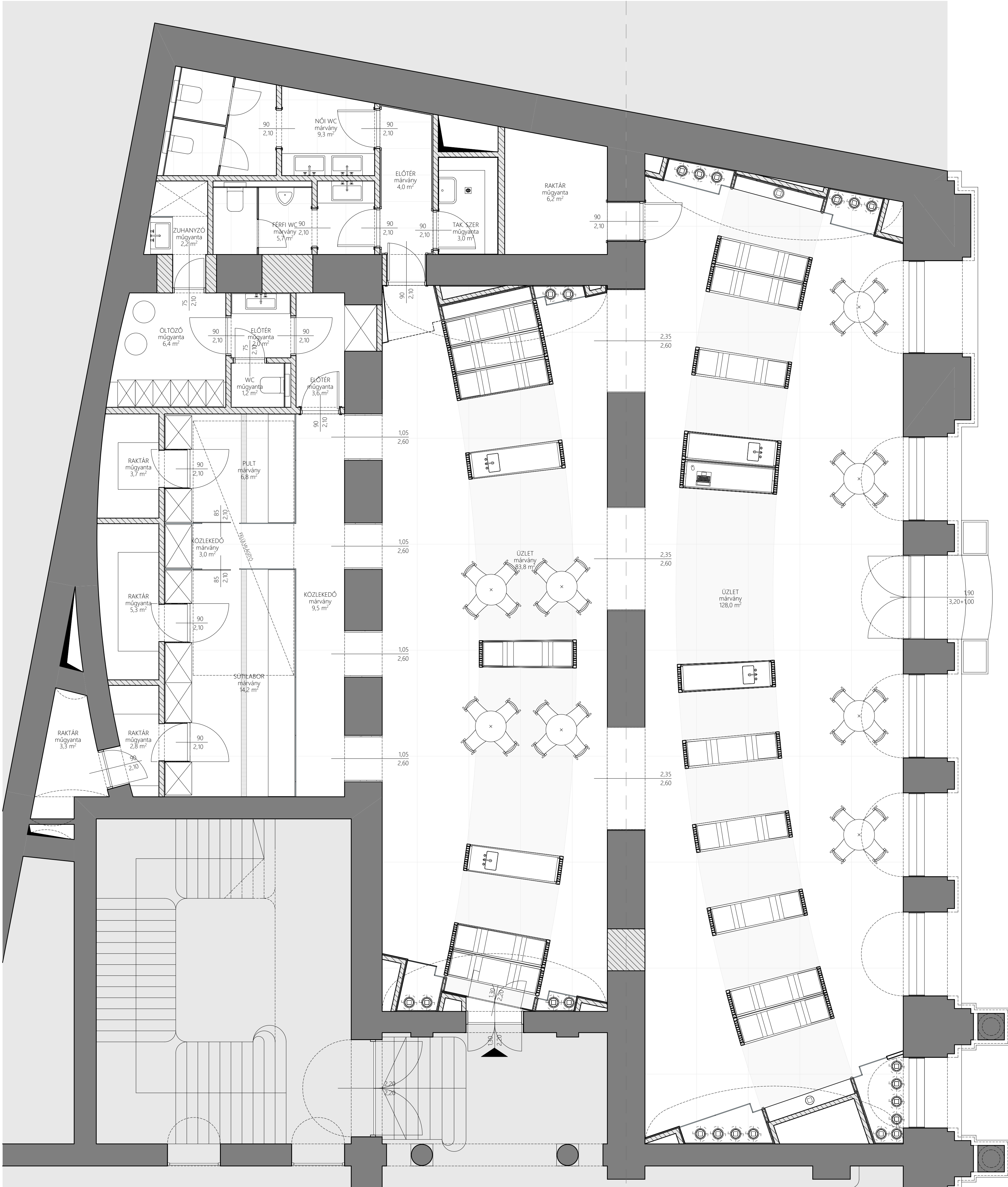
ALAPRAJZ WORKSHOP ELRENDEZÉS 1:50
