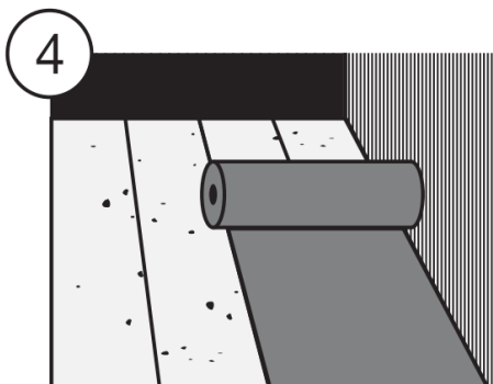
Trittschallmatte ausrollen
