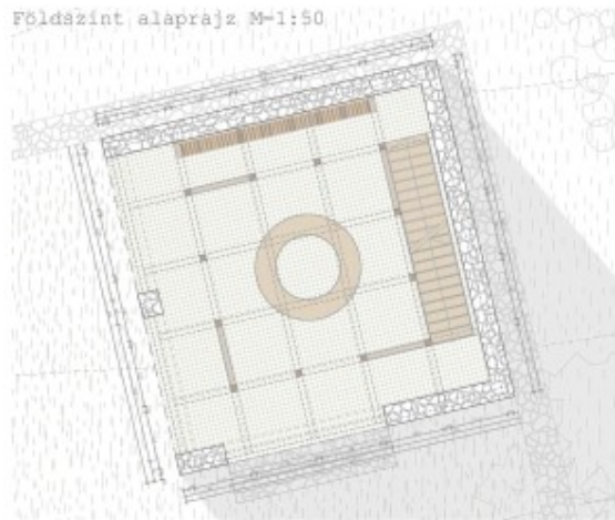
Földszint alaprajz M=1:50
