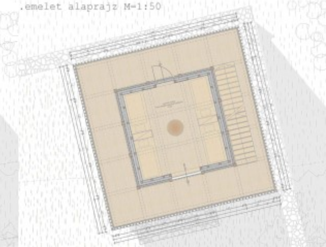
I.emelet alaprajz M=1:50
